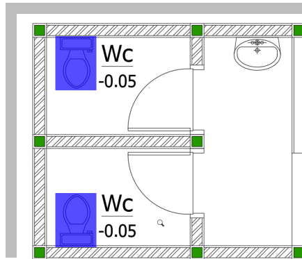
Gambar 14 , Denah Toilet Sumber: Analisis penulis, 2024
