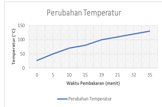
Gambar 4. 4 Grafik temperatur
