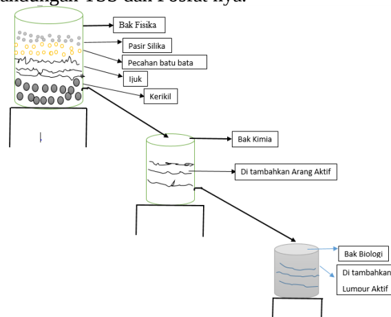
Gambar 1. Instalasi pengolahan air Limbah Detergen
